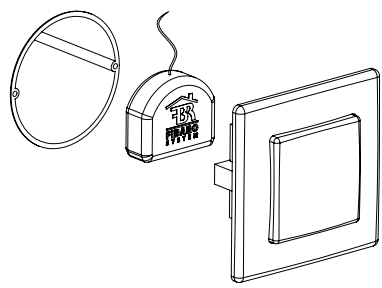
Rys.2 Montaż Łącznika Fibaro w puszcze podtynkowej.
