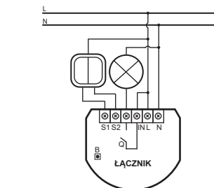
Łącznik podwójny - zasilanie napięciem sieciowym
